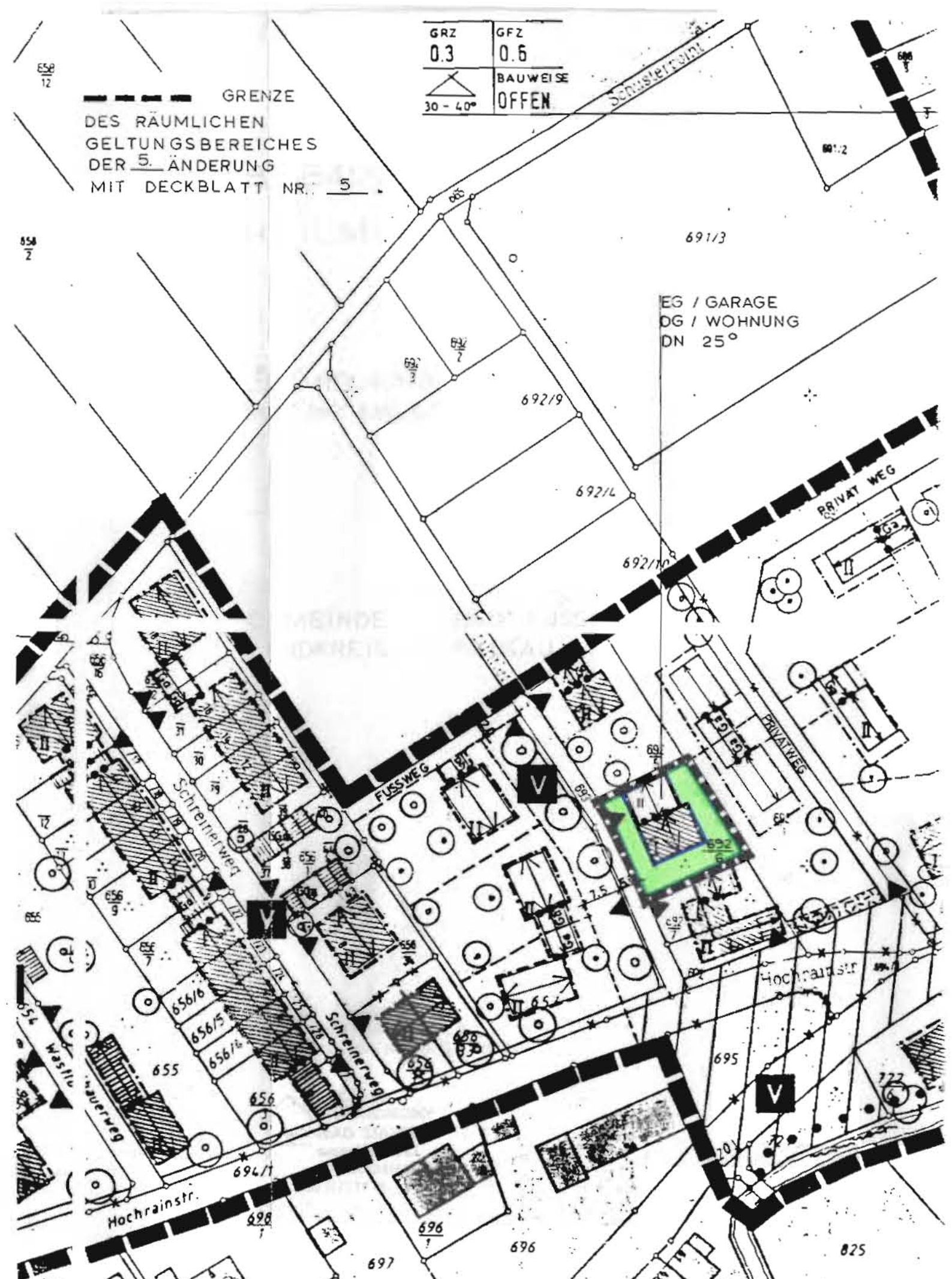
BEBAUUNGSPLAN : ÄNDERUNG
